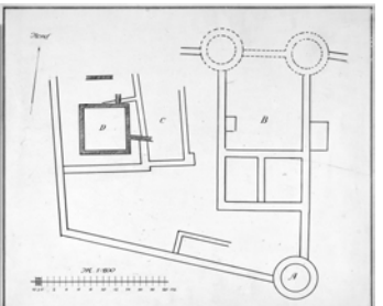
Grabungsplan der Burg von Paul Revellio aus den 1930er Jahren.
